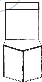
Fünfeck Theke Standard mit Aufsatzblende # 550-001-801 Maße / Angaben B/T/H 1000 x 500 x 2320 mm Gewicht: 14 kg
