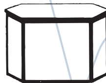
Fünfeck Theke Standard # 550-001-803 Maße / Angaben B/T/H 1280 x 560 x 905 mm Gewicht: 16 kg
